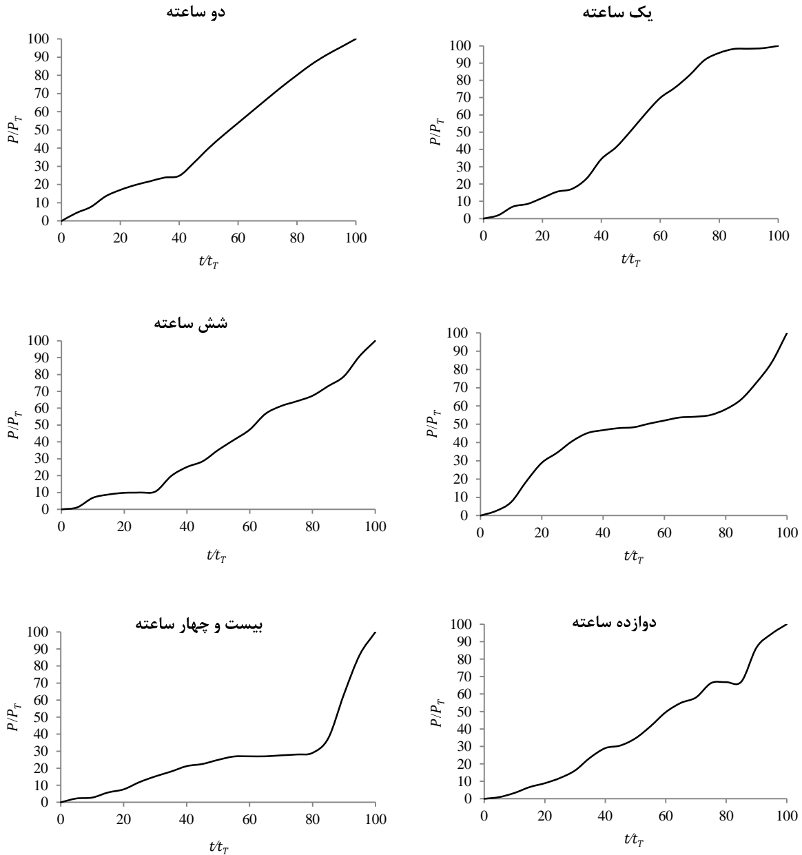
شکل ۷- نحوه تغییرات شدت بارش در طول مدت بارندگی با تداوم‌های مختلف. همان‌طور که ملاحظه می‌شود شدت بارش پس از شروع بارندگی روندی افزایشی را نشان داده و در برخی بازه‌های زمانی که شیب منحنی کاهش می‌یابد، از شدت بارش نیز کاسته می‌شود.
