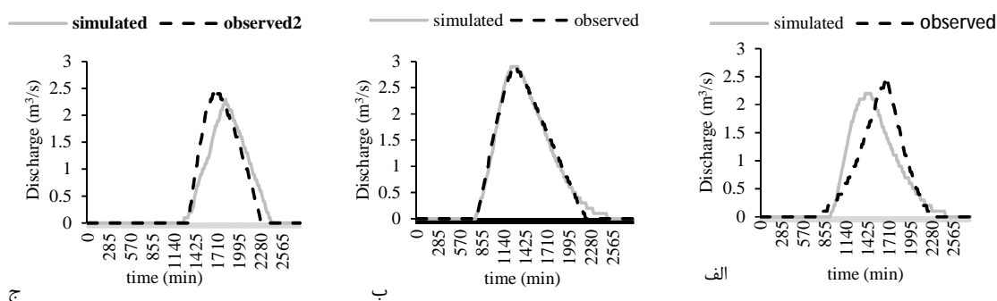
شکل ۳- آب نمود وقایع الف) ۱۳۹۱/۰۸/۲۴ ب) ۱۳۷۶/۰۱/۱۶ ج) ۱۳۷۳/۰۸/۱۶. این نمودارها پیش‌بینی قابل قبولی از میزان دبی اوج سیلاب و زمان رسیدن به آن ارائه می‌دهند؛ به طوری که اختلاف دبی اوج هیدروگراف مشاهده‌ای و شبیه‌سازی شده همواره حدود ۱۰ درصد است. تغییر و نوسان فاکتورها و عوامل مؤثر بر میزان تولید رواناب در سیلاب‌های مختلف، باعث ایجاد اختلاف در دبی، حجم رواناب و زمان رسیدن به دبی اوج می‌شود.
