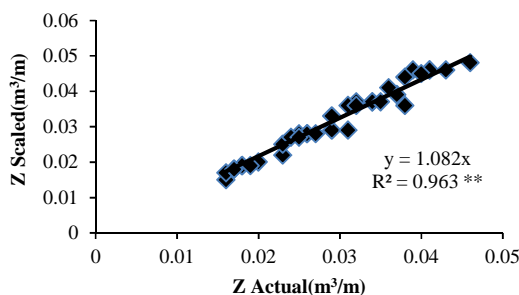
شکل ۵- نتایج رگرسیونی مقادیر نفوذ جمع‌ی اندازه‌گیری شده و تعیین شده با روش شاخص مقیاس در بافت لومی (زمان ۵۰ تا ۲۰۰ دقیقه)
