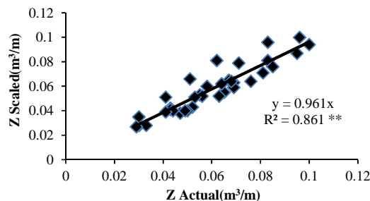
شکل ۶- نتایج رگرسیونی مقادیر نفوذ جمع‌ی اندازه‌گیری شده و تعیین شده با روش شاخص مقیاس در بافت لومی (زمان ۵۰ تا ۲۰۰ دقیقه)
