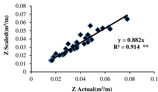
شکل ۴- نتایج رگرسیونی مقادیر نفوذ جمع‌ی اندازه‌گیری شده و تعیین شده با روش شاخص مقیاس در بافت رسی سیلتی (زمان ۵۰ تا ۲۰۰ دقیقه)
