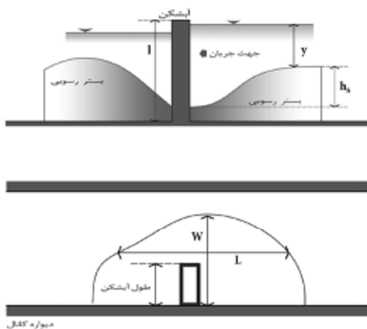
شکل ۵- نمایش شماتیک ابعاد چاله آبشستگی (پلان)
