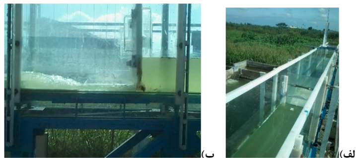
شکل ۲- الف) تصویری از فلوم حین انجام آزمایش؛ و ب) نیمرخ پرش هیدرولیکی ایجادشده در فلوم روی بستر زبر نصب شده بعد از درپچه کشویی حین انجام آزمایش
