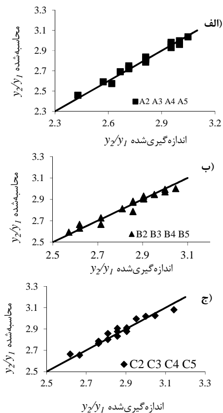
شکل ۸- مقایسه عمق نسبی به دست آمده از رابطه و عمق نسبی اندازه گیری شده برای بسترهای زیر مختلف. (الف) بستر A2 A3 A4 A5؛ (ب) بستر B2 B3 B4 B5؛ (ج) بستر C2 C3 C4 C5
