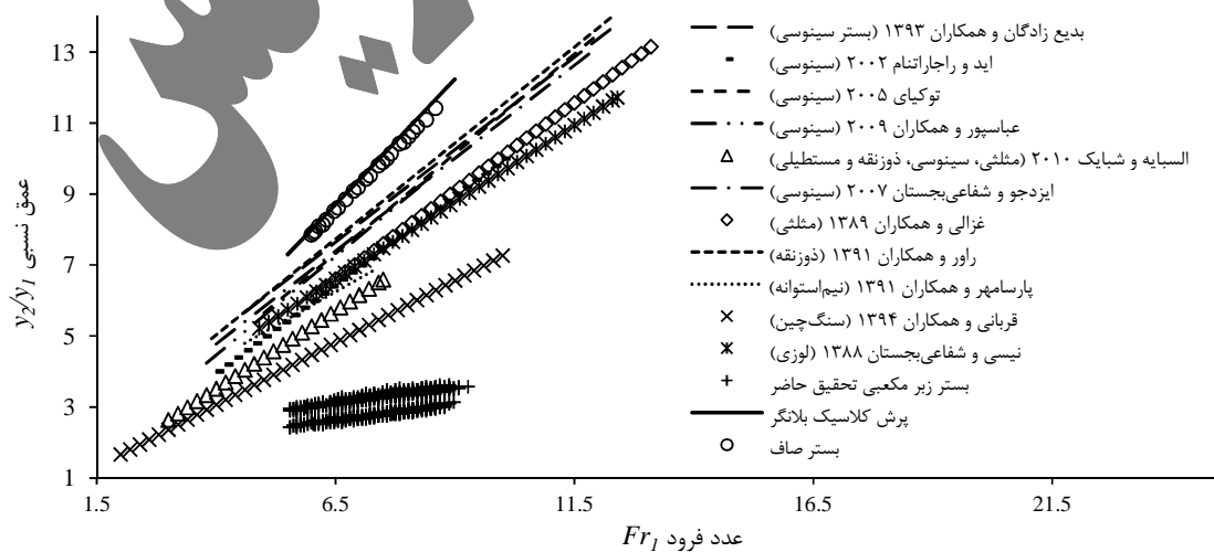
شکل ۹- مقایسه عمق نسبی پرش در مقابل عدد فرود در مطالعه حاضر و سایر تحقیقات انجام شده
