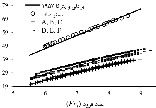
شکل ۶- مقادیر \frac{L_j}{y_1} در مقابل Fr_1 در آرایش زیگزگی، ردیفی و بستر صاف
