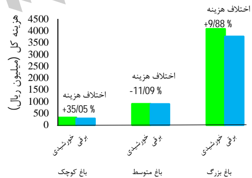
شکل ۲- هزینه موردنیاز برای پمپاژ خورشیدی نسبت به پمپاژ برقی در باغ پسته با نرخ بهره ۱۰ درصد
