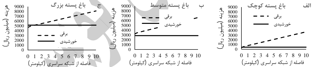
شکل ۷- مقایسه هزینه سیستم پمپاژ برقی و خورشیدی باغ پسته (الف: کوچک، ب: متوسط و ج: بزرگ) در فواصل مختلف از شبکه سراسری توزیع برق
