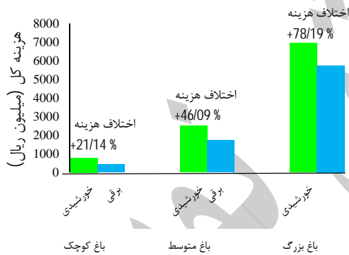
شکل ۳- هزینه موردنیاز برای پمپاژ خورشیدی نسبت به پمپاژ برقی در باغ بادام با نرخ بهره ۵ درصد
