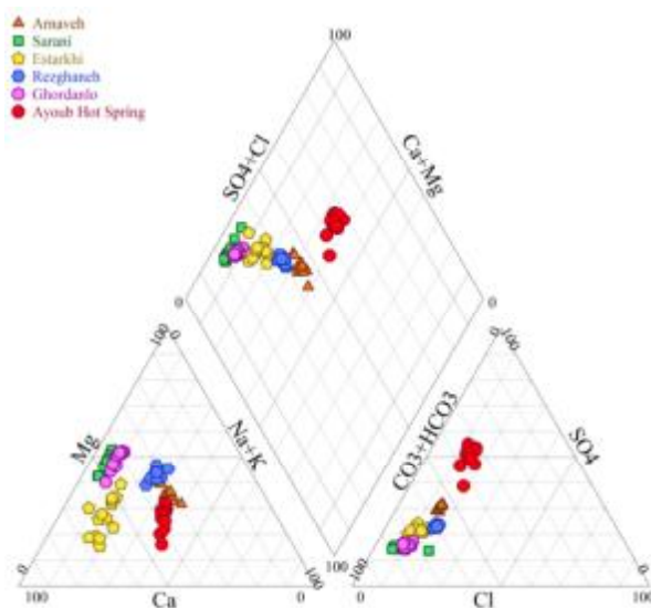
شکل ۲- نمودار پایپر چشمه‌های کارستی مهم مورد مطالعه در استان خراسان شمالی
