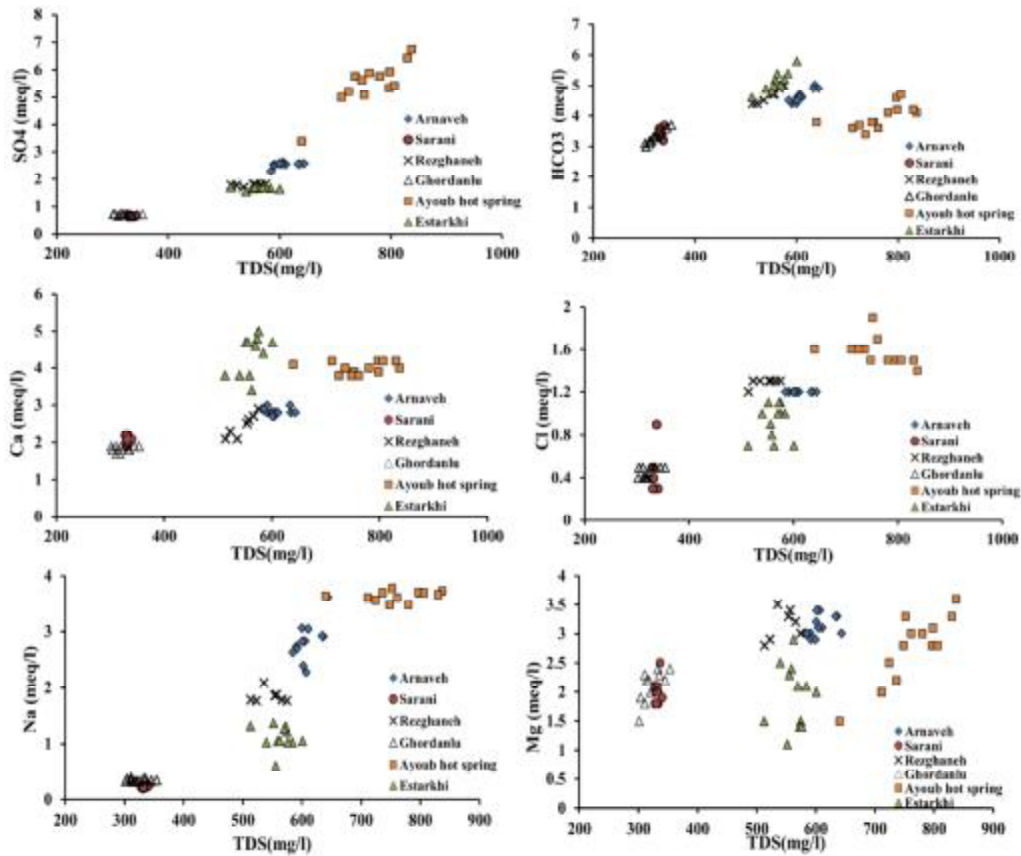
شکل ۴- نمودار TDS در برابر کاتیون‌ها و آنیون‌های اصلی نمونه‌های آب چشمه‌های مورد مطالعه
