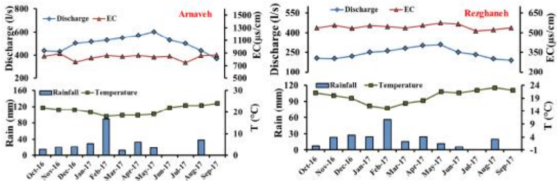
شکل ۵- بررسی پارامترهای فیزیکو- شیمیایی چشمه‌های مورد مطالعه
