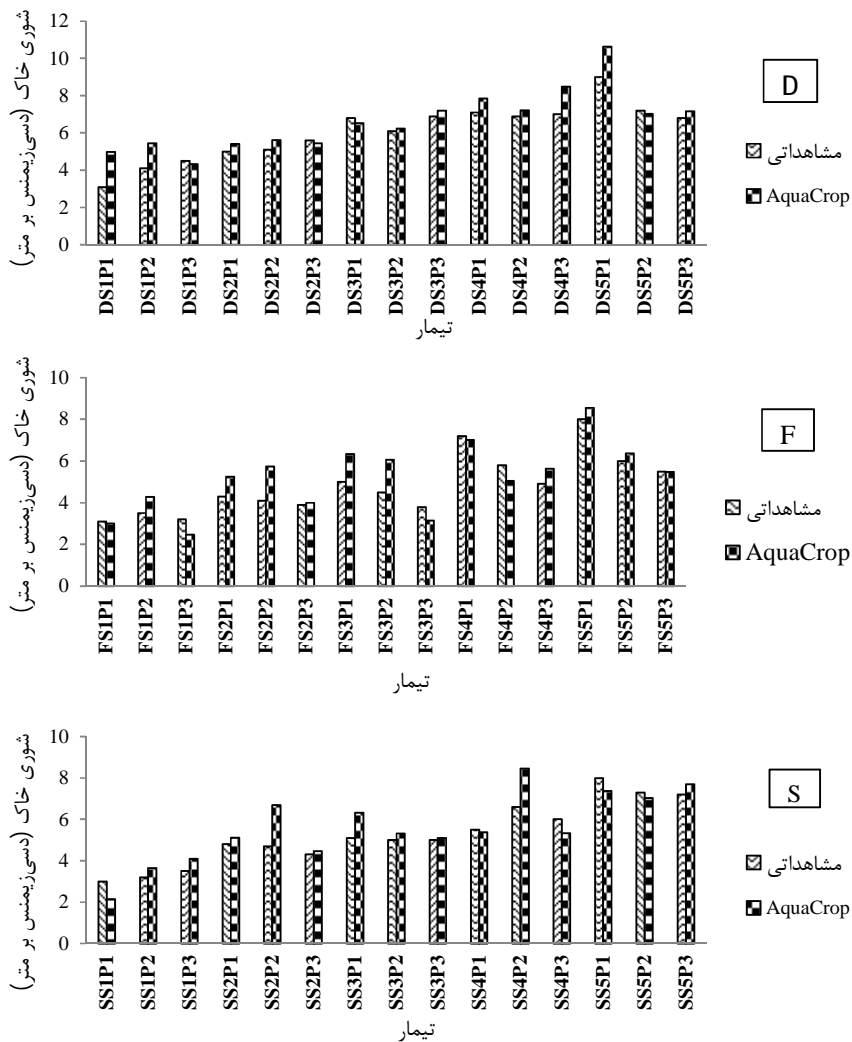
شکل ۵- مقایسه نتایج شوری خاک مشاهداتی و شبیه‌سازی‌شده با استفاده از مدل AquaCrop (D, F, S) به‌ترتیب آبیاری بارانی با آب شور، آبیاری بارانی با تلفیق آب شور و شیرین و آبیاری سطحی؛ S1, S2, S3, S4 و S5 به‌ترتیب، شوری آب آبیاری به میزان ۳/۲، ۳/۵، ۴/۶، ۵/۱ و ۵/۱ دسی‌زیمنس بر متر و P1, P2 و P3 به‌ترتیب، عمق ۱۵، ۴۵ و ۷۵ سانتی‌متر است.
