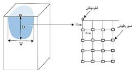
شکل 4- شمایی از محل قرارگیری قطره‌چکان و سنسورهای رطوبتی داخل جعبه آزمایشگاهی
