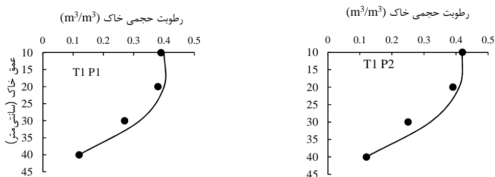
شکل ۶- مقایسه توزیع رطوبت خاک برآوردی (خط ممتد) توسط مدل عددی HYDRUS-2D و مشاهداتی (نقاط توپر) در تیمارهای مختلف 72 ساعت پس از شروع آبیاری
