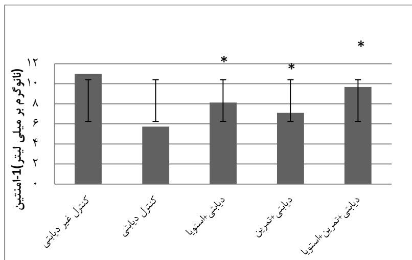
نمودار ۶. میانگین آمینتین-۱ در گروه‌های مورد مطالعه
