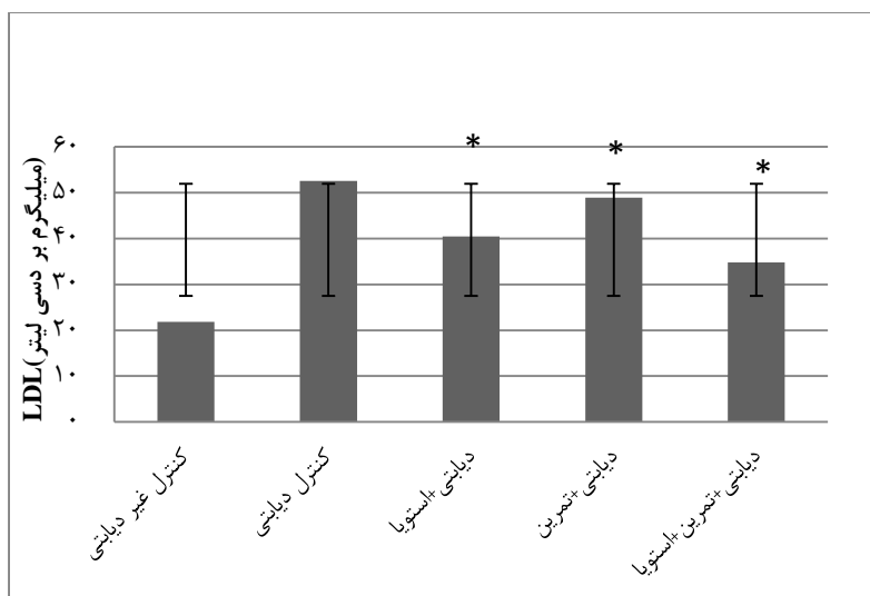
نمودار ۳. میانگین LDL در گروه‌های مورد مطالعه
