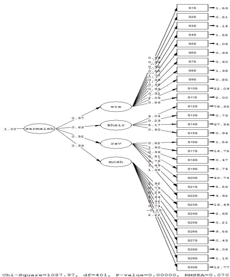
شکل ۲. تحلیل عاملی تائیدی سرمایه اجتماعی (خروجی لیزرل)
