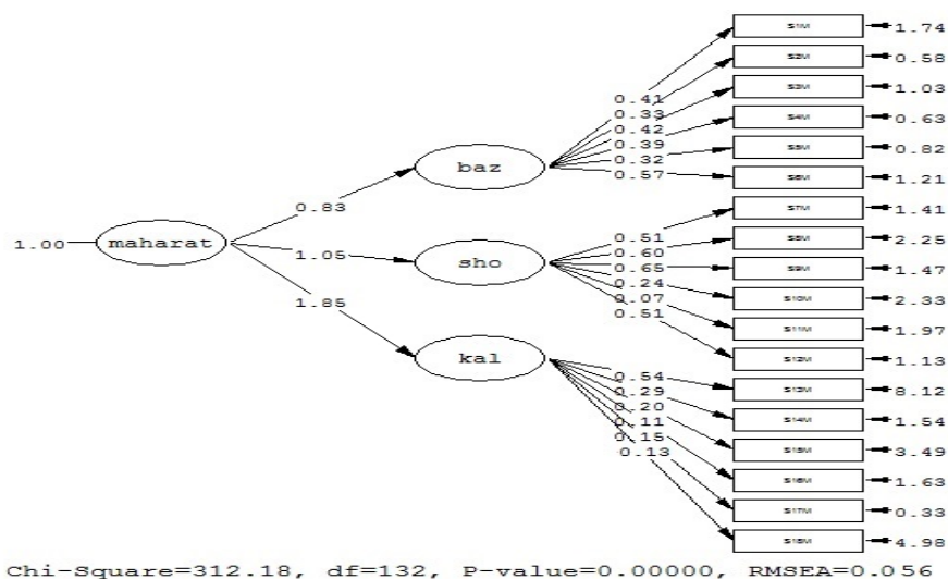
شکل ۱. تحلیل عاملی تأییدی مهارت‌های ارتباطی (خروجی لیزرل)
