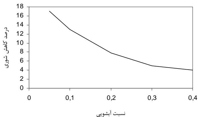
شکل ۳- شبیه سازی مدل watsuit - درصد کاهش غلظت نمک در محلول خاک در اثر فرایند تشکیل رسوب و رابطه آن با جزء آبیاری
