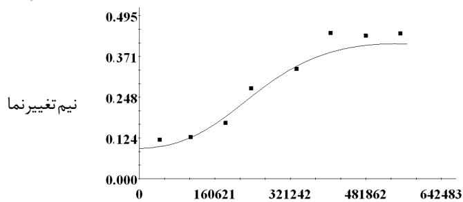
شکل 3- نیم تغییرنمای تناخص فرساینده‌گی
