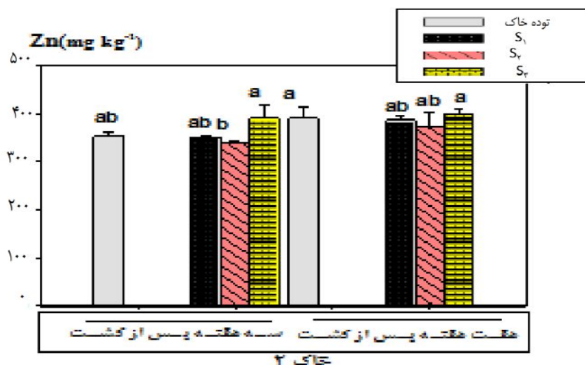
(ت) - میانگین غلظت روی قابل استخراج با \text{HNO}_3 ( \text{mg kg}^{-1} ) شکل 3- تغییر زیست فراهمی روی در مناطق مختلف جداسازی شده خاک ( S_1, S_2, S_3 ) سه و هفت هفته پس از کشت برای عصاره گیرهای مختلف (تفاوت معنی‌داری در سطح پنج درصد می‌باشد)
