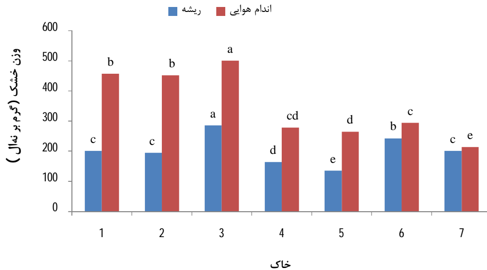
شکل 2- میانگین وزن خشک اندام هوایی و ریشه نارنگی انشو میاگاوا با پایه سوینگل سیتروملو در خاک‌های مختلف (میانگین‌های مربوط به هر ستون که دارای حروف لاتین مشترک هستند در سطح احتمال پنج درصد تفاوت معنی‌داری با یکدیگر ندارند)
