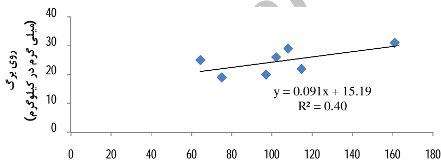
روی ریشه (میلی گرم در کیلوگرم)
