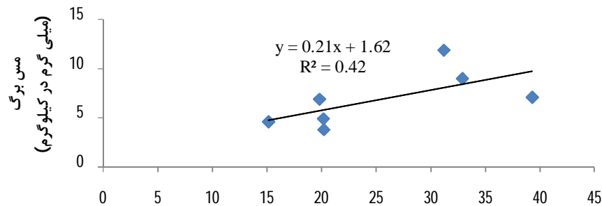
مس ریشه (میلی گرم در کیلوگرم)
