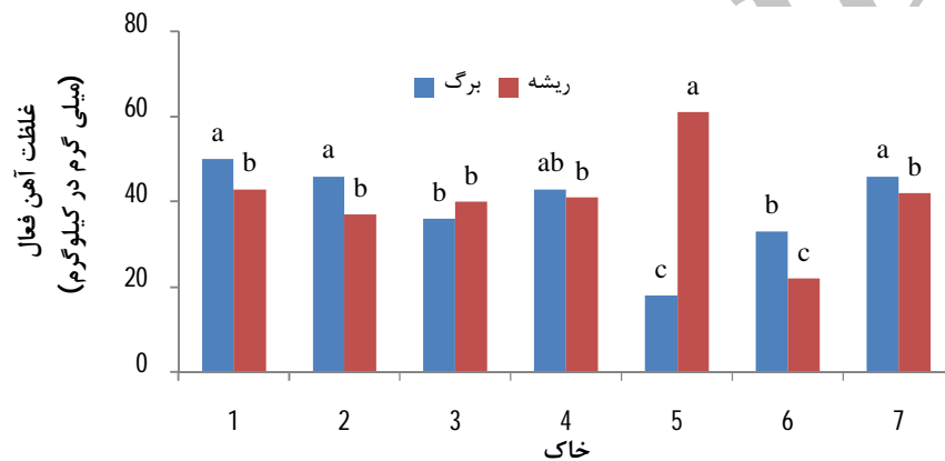
شکل 6- میانگین غلظت آهن فعال برگ و ریشه نارنگی انشو میاگاوا با پایه سوینگل سیتروملو در خاک‌های مختلف (میانگین‌های مربوط به هر ستون که دارای حروف لاتین مشترک هستند در سطح احتمال پنج درصد تفاوت معنی‌داری با یکدیگر ندارند)
