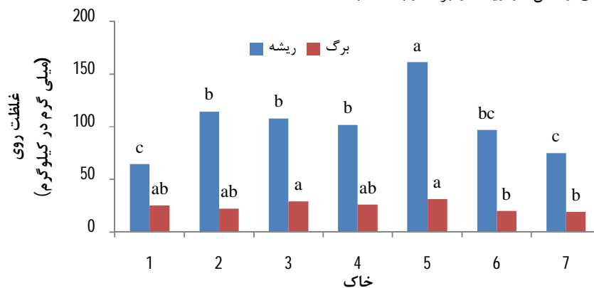
شکل 8- میانگین غلظت روی برگ و ریشه نارنگی انشو میاگاوا با پایه سوینگل سیتروملو در خاک‌های مختلف (میانگین‌های مربوط به هر ستون که دارای حروف لاتین مشترک هستند در سطح احتمال پنج درصد تفاوت معنی‌داری با یکدیگر ندارند)
