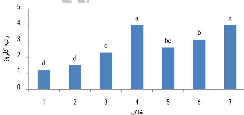
شکل 3- میانگین درجه زردی برگ نارنگی انشو میاگاوا با پایه سوینگل سیتروملو در خاک‌های مختلف (میانگین‌های مربوط به هر ستون که دارای حروف لاتین مشترک هستند در سطح احتمال پنج درصد تفاوت معنی‌داری با یکدیگر ندارند)
