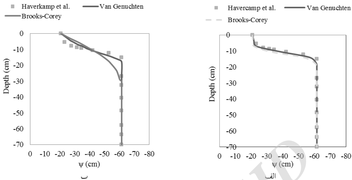
شکل 5- پروفیل فشار محاسبه شده با استفاده از توابع وان گنوختن و بروکز-کوری (الف) مدل حاضر (ب) مدل عزیز پور و محمودیان شوشتری (2012)
