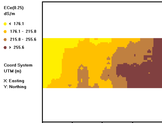
شکل 6- نقشه شوری خاک پیش‌بینی شده خروجی نرم‌افزار با استفاده از معادله واسنجی انتخاب شده در سه عمق مورد بررسی الف) 0/05 cm، ب) 0/15 cm و ج) 0/25 cm
