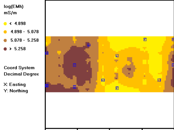
شکل 4- محل‌های نمونه‌برداری انتخاب شده به عنوان خروجی از برنامه ESAP-RSSD از داده‌های پیمایش شده
