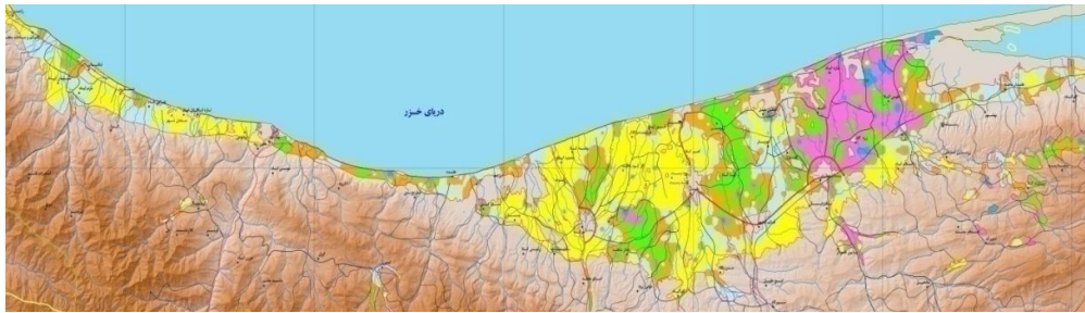
شکل 2- پراکنش کربنات کلسیم در خاک‌های استان مازندران. مناطق با رنگ زرد، 0-5 درصد؛ آبی کم‌رنگ، 5-10 درصد؛ قهوه‌ای، 10-15 درصد؛ سبز، 15-20 درصد؛ صورتی، 20-30 درصد؛ آبی پررنگ، 30-50 درصد و خاکستری، بیش از 50 درصد کربنات کلسیم معادل را نشان می‌دهند (طهرانی و همکاران، 1390).
