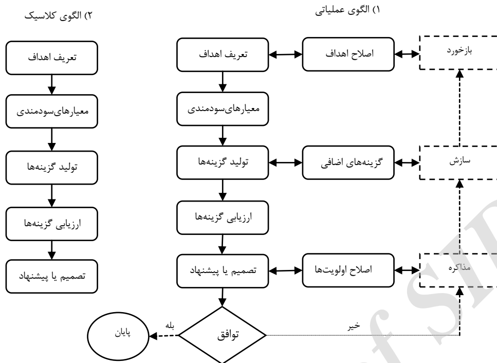
شکل ۱- ساختار عملیاتی و کلاسیک شبیه‌سازی مربوط به تحلیل سیستم‌های منابع آب (لاکس و ون بیک، ۱۳۹۲).
