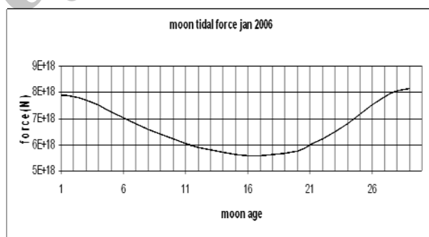
شکل ۴- نیروی کشند قمری از روز ۲۴۵۳۳۷۵/۵ تا روز ۲۴۵۳۷۶۶/۵ تقویم ژولین
