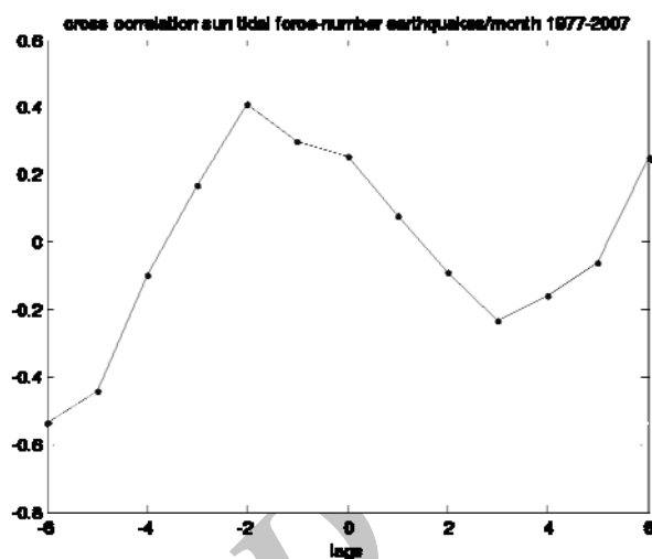
شکل ۸- نمودار همبستگی متقابل بین نیروی کشند خورشیدی و بسامد ماهانه زمینلرزه‌ها از ۱۹۷۷ تا ۲۰۰۷
