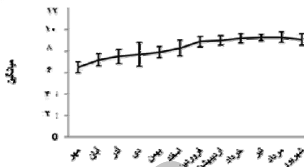
نمودار ۶ - ارتباط بین میانگین عرض کاراپاس با ماه‌های سال در جنس نر (میانگین \pm خطای معیار)
