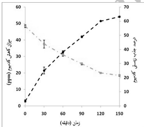
شکل ۴- منحنی حذف فلز کادمیوم در غلظت ۵۰ میلی گرم بر لیتر در دمای ۳۰°C و سرعت ۱۶۰ rpm
