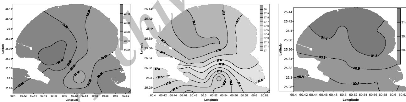
شکل ۲: منحنی‌های هم‌تراز دما، شوری و چگالی به ترتیب از راست به چپ در شهریور ماه
