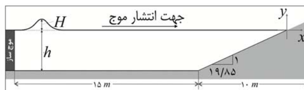
شکل ۱: طرح کانال آزمایش برای تولید و انتشار موج تنها بر اساس مشخصات مرجع (Synolakis, 1987)
