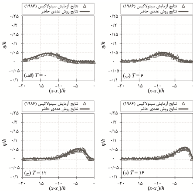
شکل ۸: مقایسه نتایج شبیه‌سازی عددی تغییرات سطح آزاد سیال در کانال موج برای نسبت ارتفاع موج به عمق آب H/h = 0.04 و h = 0.2855
