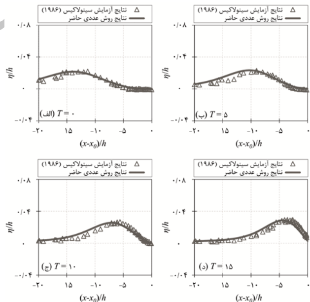
شکل ۹: مقایسه نتایج شبیه‌سازی عددی تغییرات سطح آزاد سیال در کانال موج برای نسبت ارتفاع موج به عمق آب H/h = 0.02 و h = 0.3097
