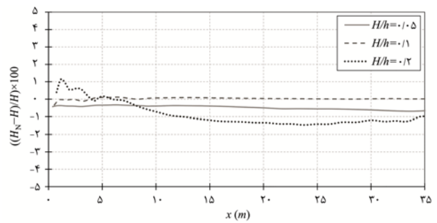
شکل ۷: انتشار موج تنها در کانال‌های طولی با استفاده از روش عددی مورد نظر
