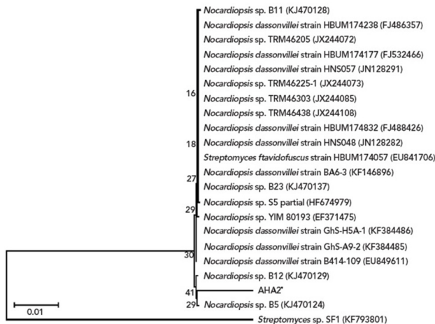
شکل ۳: درخت فیلوژنی به روش پیوند همجواری ۲ گونه AHA2 بر اساس توالی ژن 16S rDNA، Streptomyces sp. SF(KF793801)، به عنوان برون گروه انتخاب شده است.
