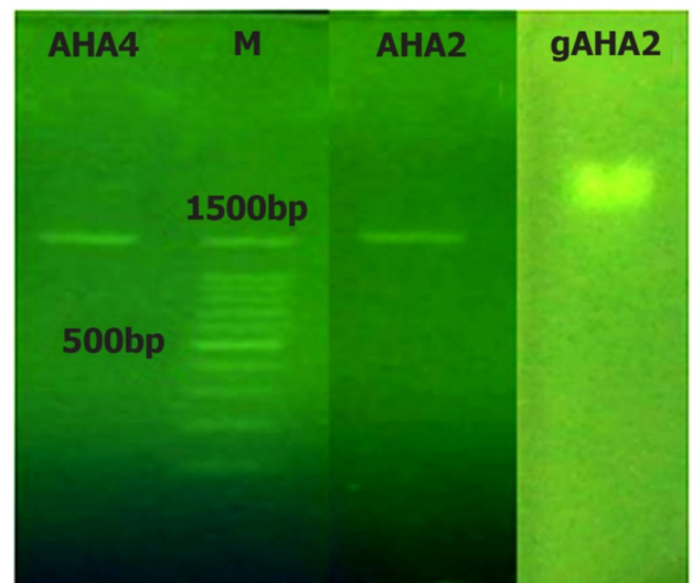
شکل ۲: ژل الکتروفورز: gAHA2 نشان‌دهنده باند حاصل از استخراج DNA ژنومی از ایزوله AHA2، AHA2 محصول PCR ژن 16S rRNA (در محدوده ۱۵۰۰ جفت بازی) است. M: مارکر ۱۰۰ جفت بازی DNA
