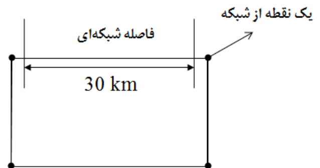
شکل ۱: فاصله شبکه‌ای و نقاط شبکه‌ای در حالت مرجع
