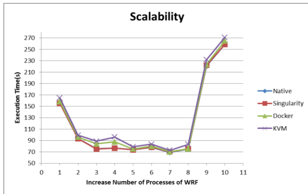
شکل ۳: نمودار مقایسه مقیاس‌پذیری اجرای مدل در محیط‌های عملیاتی با افزایش تعداد پردازش‌های موازی و هم‌زمان
