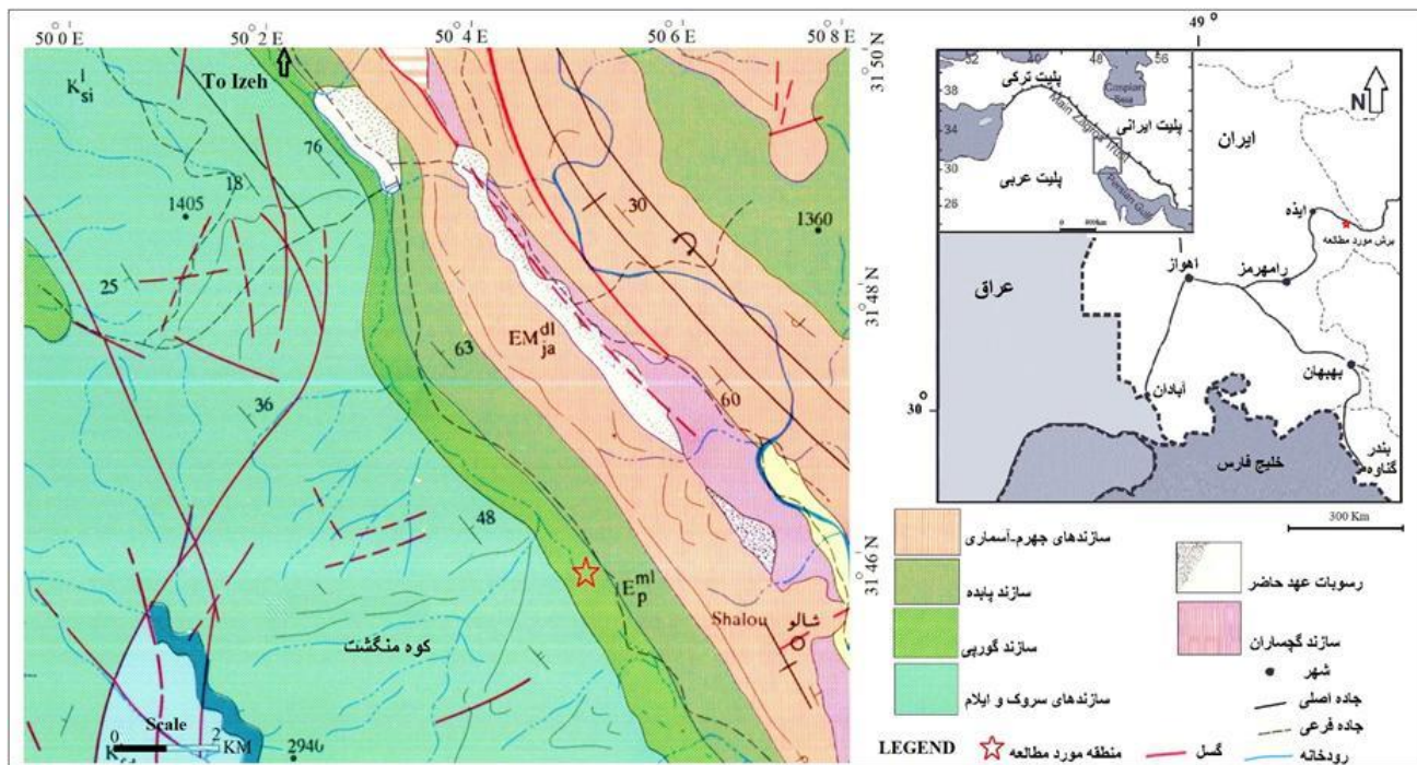
شکل ۱: راه دسترسی و موقعیت ناحیه مورد مطالعه در جنوب خاور ایذه، برش مطالعه شده در نقشه زمین شناسی که توسط ستاره مشخص شده است (برگرفته شده از نقشه زمین‌شناسی ۱:۱۰۰۰۰۰ دهلز، سازمان زمین‌شناسی کشور).
