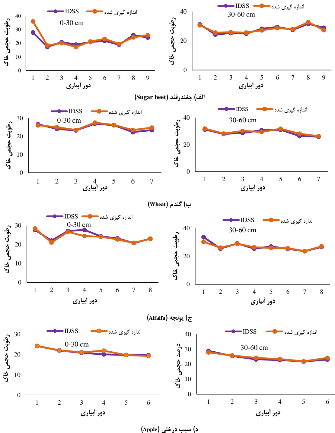
شکل ۱۲- مقایسه مقادیر رطوبت خاک اندازه‌گیری شده و شبیه‌سازی شده توسط IDSS (الف تا د) Figure 12- Comparison of soil moisture values measured and simulated by IDSS (a-d)
