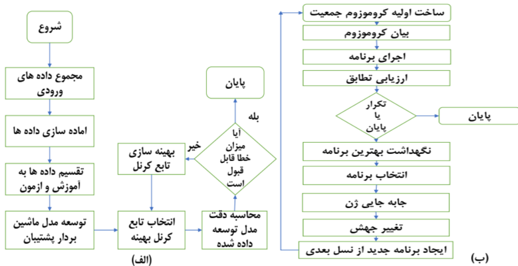
شکل ۲- مراحل اجرای ماشین بردار پشتیبان (SVM) (الف) و برنامه‌ریزی بیان ژن (GEP) (ب) Figure 2- Implementation steps of support vector machine (SVM) (a) and gene expression programming (GEP) (b)
