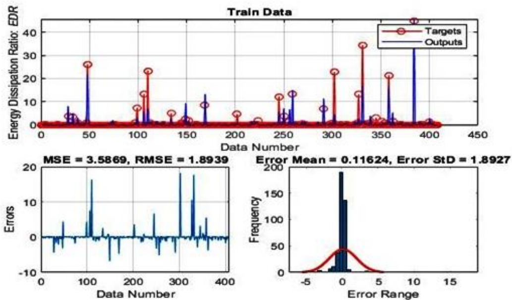
شکل ۱۵- نتایج خروجی مدل GMDH در محیط متلب در مرحله آموزش در ایستگاه حسن‌آباد Figure 15- The output results of the GMDH model in the MATLAB environment during the training phase in Hasan Abad station
