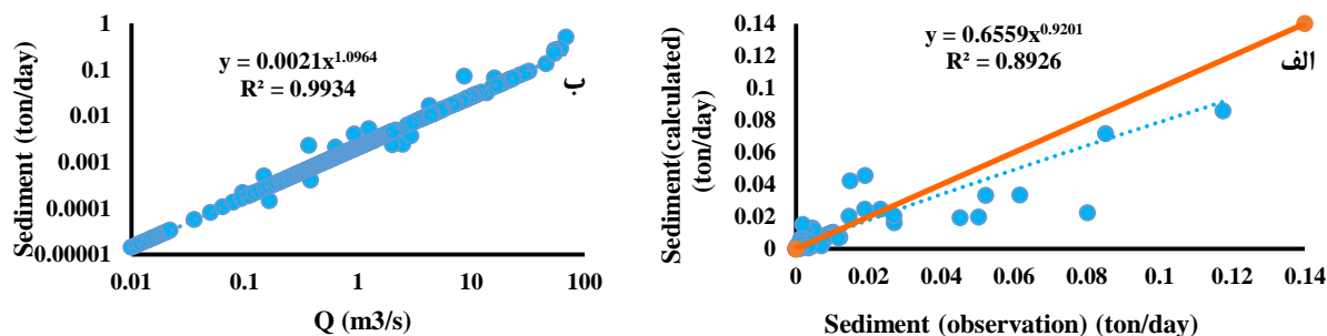
شکل ۷- منحنی سنجه رسوب قسمت آموزش (الف) و مقادیر محاسباتی و مشاهداتی برای قسمت آزمون (ب) Figure 7- Sediment gauge curve for the training part (a) and calculated and observed values for the test part (b)
