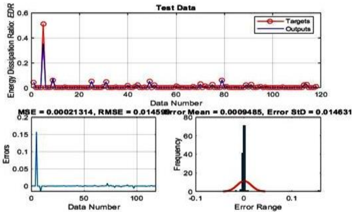
شکل ۱۴- نتایج خروجی مدل GMDH در محیط متلب در مرحله آموزش در ایستگاه حسن‌آباد Figure 14- The output results of the GMDH model in the MATLAB environment during the training phase in Hasan Abad station
