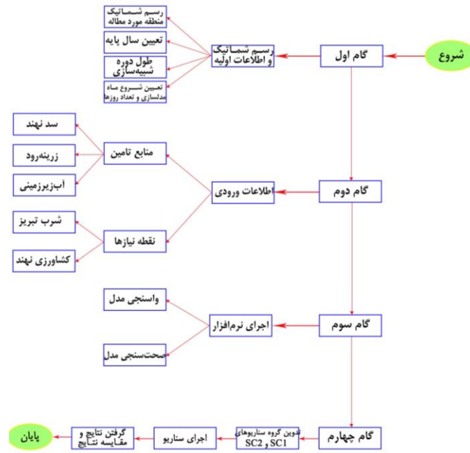
شکل ۷- نمای کلی مدل شبیه‌سازی سد نهند Figure 7- Overview of the simulation model of Nahand Dam
