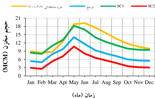
شکل ۱۰- مقایسه مقادیر متوسط حجم ماهانه مخزن سد نهند برای دوره ۲۰۲۱-۲۰۴۰ نسبت به دوره مشاهداتی (۲۰۰۰-۲۰۲۰) تحت سناریوهای تدوین شده در مدل WEAP Figure 10- Comparison of the average monthly volume of the Nahand Dam reservoir for the period of 2021-2040 compared to the observation period (2000-2020) under the scenarios developed in the WEAP model
