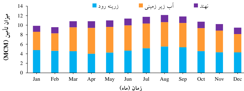
شکل ۳- میزان تأمین ماهانه هر یک از منابع تأمین برای سال پایه (۲۰۱۶) در منطقه مورد مطالعه Figure 3- The amount of monthly supply of each supply source for the base year (2016) in the study area
