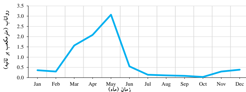
شکل ۴- رواناب رودخانه نهند در سال پایه (۲۰۱۶) Figure 4- Nahand River runoff in the base year (2016)
