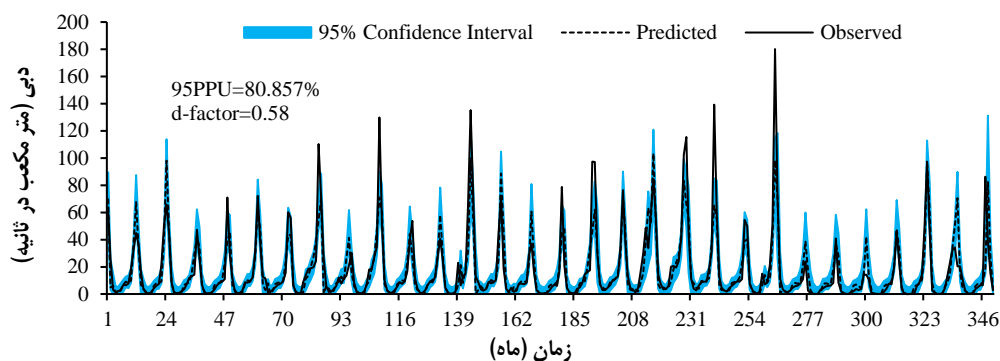
شکل ۸- مقادیر مشاهداتی و پیش بینی شده حاصل از مدل ANN و باند اطمینان ۹۵ درصد در مرحله آموزش Figure 8- The observed and predicted values obtained from the ANN model and the 95% confidence interval in the training phase
