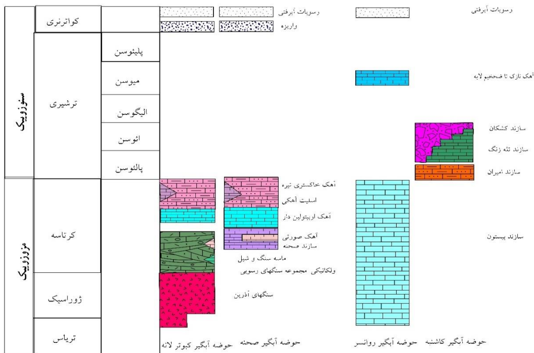
شکل ۸- مقایسه ستون چینه‌شناسی حوضه‌های آبخیز
