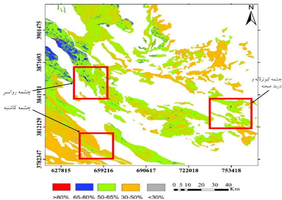
شکل ۳- نقشه نهایی برآورد تغذیه در منطقه مطالعه شده
