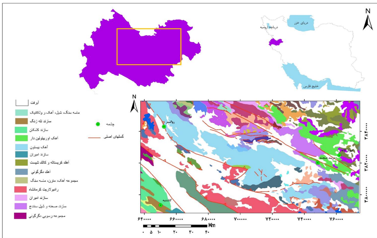
شکل ۱- موقعیت جغرافیایی و نقشه زمین‌شناسی چشمه‌های مطالعه‌شده
