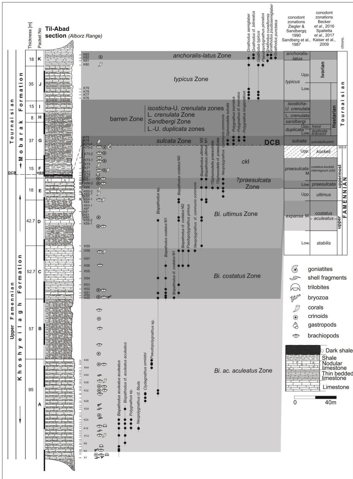
شکل ۵- ستون سنگ‌چینه‌ای، بایوزون‌ها و پراکندگی کنودونتها در برش تیل‌آباد
