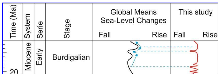
شکل ۱۶- انطباق نمودار نوسان‌های نسبی سطح آب دریا در برش مطالعه‌شده با نمودار جهانی (برگرفته از Haq and Al-Qahtani 2005)
