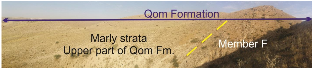
شکل ۴- مرز تدریجی بین توالی‌های مارنی بخش بالایی سازند قم با توالی‌های کربناته ضخیم‌لایه عضو F سازند قم (دید به سمت جنوب)
