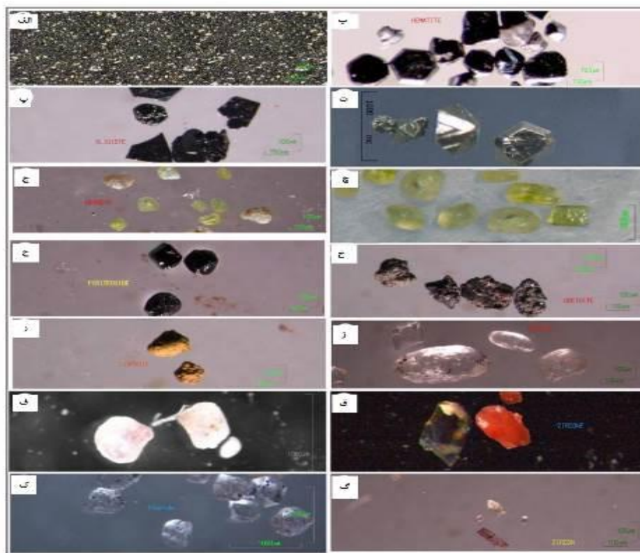
شکل ۹- کانی‌های سنگین شناسایی شده در رسوبات جزیره هرمز: الف. مگنتیت، ب. هماتیت، پ. الیژیست، ت. هماتیت، مارتیت، الیژیست، ج. اپیدوت، چ. پیروکسن، ح. پیریت، خ. گوتیت، ر. لیمونیت، ز. آپاتیت، ف. باریت، ق. زیرکن، ک. فلوریت، گ. زیرکن
