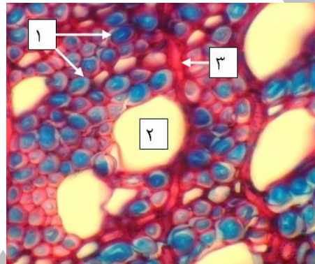
شکل ۱- مقطع عرضی قسمت دارای بیشترین تنش. مقیاس: میلی‌متر 10=50 میکرون. ۱: فیبرهای ژلاتینی آبی شده که نشان‌دهنده تشکیل چوب کشتی اند، ۲: آوند، ۳: اشعه چوبی.
