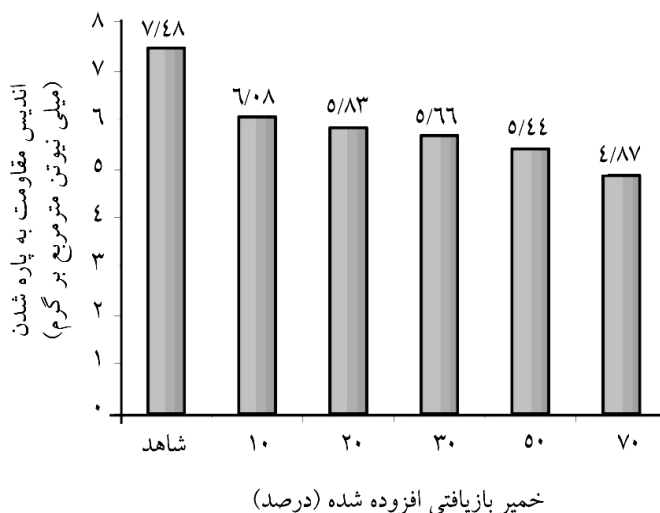
شکل ۲- تغییرات تندیس مقاومت به پاره شدن کاغذهای دست‌ساز بر اثر تغییر مقدار خمیر بازیافتی.
