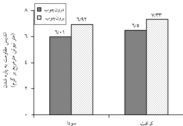
شکل ۴- مقایسه شاخص مقاومت به پاره شدن درون چوب و برون چوب خمیر سودا و کرافت.
