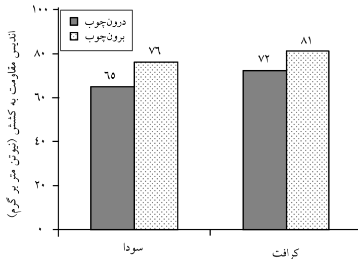
شکل ۳- مقایسه شاخص مقاومت به کشش درون چوب و برون چوب خمیر سودا و کرافت.
