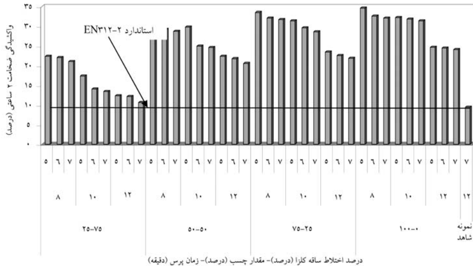
شکل ۴- تأثیر متقابل درصد اختلاط ساقه کلزا با خرده‌چوب، مقدار چسب و زمان پرس روی واكشیدگی ضخامت ۲ ساعت غوطه‌وری در آب.
