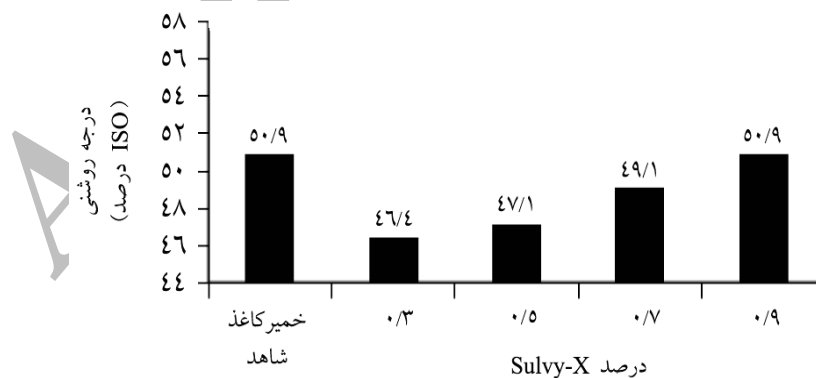
شکل ۱- تأثیر Sulvy-x بر درجه روشنی خمیرهای کاغذ روزنامه بازیافتی.
