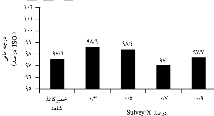
شکل ۳- تأثیر Sulvy-x بر درجه ماتی خمیرهای کاغذ روزنامه بازیافتی.
