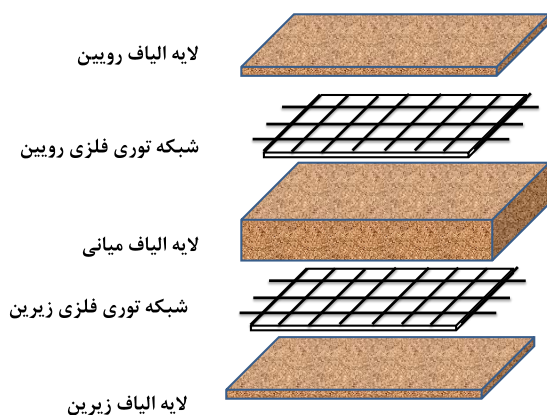
شکل 1- شیوه قرار گرفتن لایه‌ها و شبکه‌های تقویت کننده
