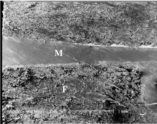
شکل 4- تصویر میکروسکپ الکترونی از سطح اتصال شبکه‌های فلزی با الیاف؛ الف: شبکه آغشته شده به چسب اپوکسی پیوستگی همه جانبه فلز با چسب اپوکسی درون تخته را نشان می‌دهد؛ ب: شبکه فلزی بدون آغشتگی اولیه که می‌توان خط فاصله بین رشته و الیاف را دید؛ M: فلز؛ F: الیاف
