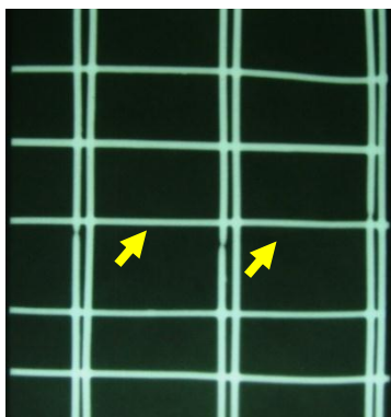
شکل 3- نواحی شکست رشته‌های تقویت‌کننده در آزمون خمش: رشته‌های شبکه زیرین که تحت کشش قرار داشته‌اند، دچار شکست شده‌اند
