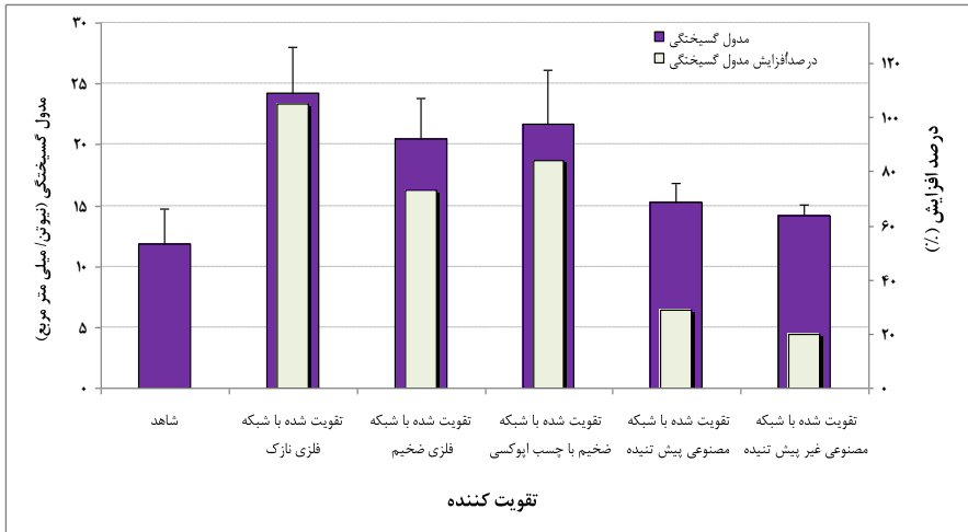
شکل 2- میانگین مدول‌های الاستیسیته (الف) و گسیختگی (ب) تخته‌ها و درصد افزایش آن
