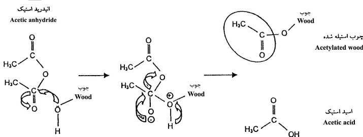
شکل ۱- مکانیسم واکنش انیدریداستیک با چوب طی فرآیند استیله کردن (مجبی، ۲۰۰۳).
