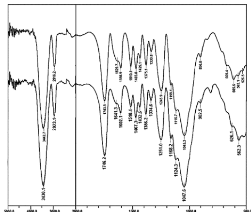
شکل ۳- طیف FTIR نمونه‌های استیل ۵ درصد (بالا: هوازده، پائین: هوازده)
