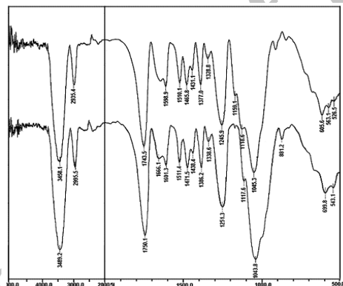
شکل ۴- طیف FTIR نمونه‌های استیل ۹ درصد (بالا: هوازده، پائین: هوازده)
