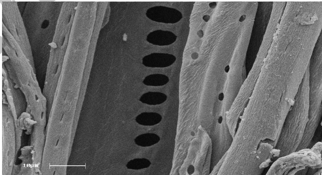
شکل ۶- تصویر میکروسکوپ الکترونی سطح شعاعی چوب راش شاهد ( 500\times )
