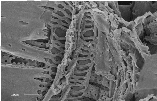
شکل ۹- تصویر میکروسکوپ الکترونی اثر هوازدگی بر سطح شعاعی چوب راش استیله (۵۰۰ X).
