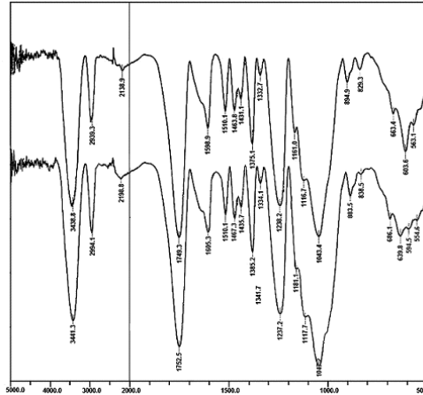
شکل ۵- طیف FTIR نمونه‌های استیله ۱۶ درصد (بالا: هوازده، پائین: هوازده)
