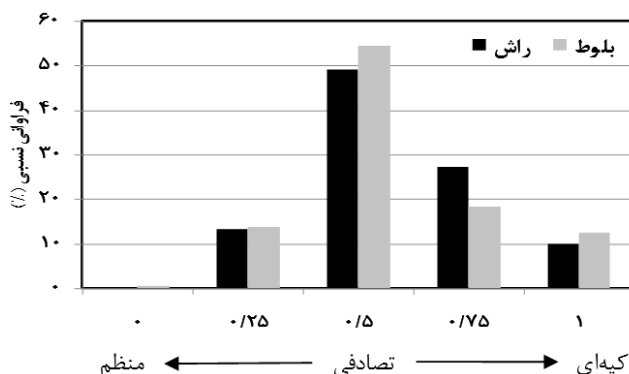
شکل ۳- توزیع ارزش‌های شاخص زاویه یکتواخت مربوط به گونه‌های راش و بلوط.
