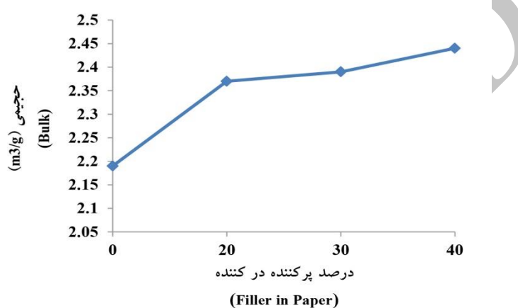
شکل ۲- تأثیر پرکننده معدنی بر حجمی کاغذ در سطوح مختلف پرکننده معدنی.
