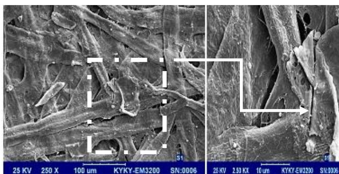
شکل ۱- تصاویر الکترونی سطوح کاغذ تیمار شده با نانو نقره.
