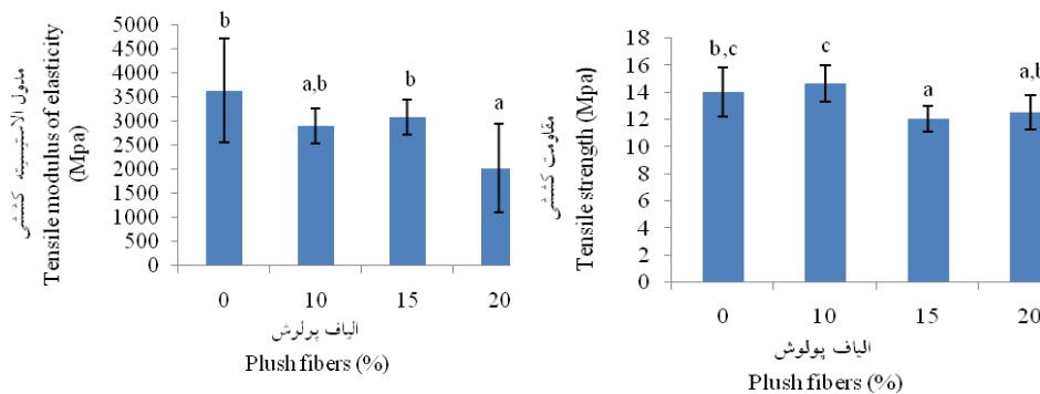
شکل ۲- اثر میزان الیاف ضایعاتی پولوش بر مدول الاستیسیته کششی و مقاومت کششی.
