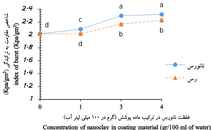
شکل ۶- تغییرات میزان شاخص ترکیب در نتیجه مصرف مقادیر مختلف رس و نانورس به‌عنوان یک عامل پوششی در کاغذ.
