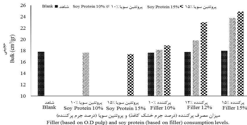
شکل ۴- تأثیر افزودن پرکننده و پروتئین سویا پیش‌اختلاط شده بر حجمی کاغذ.
