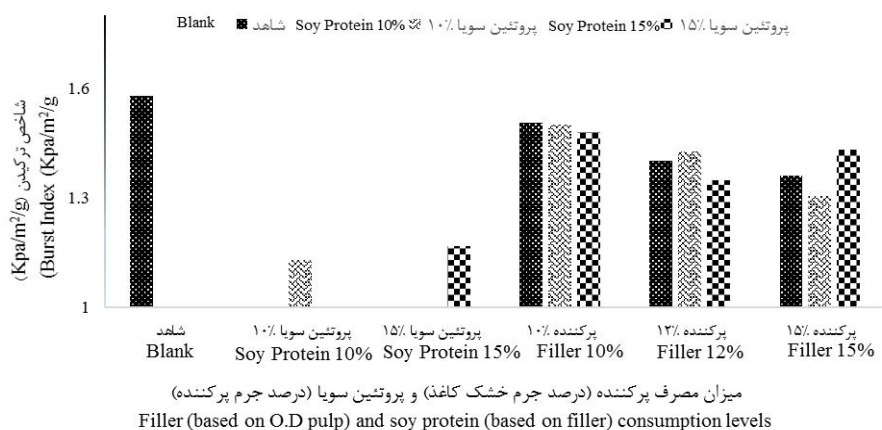
شکل ۷- تأثیر افزودن پرکننده و پروتئین سویا پیش‌اختلاط شده بر شاخص ترکیدن کاغذ.
