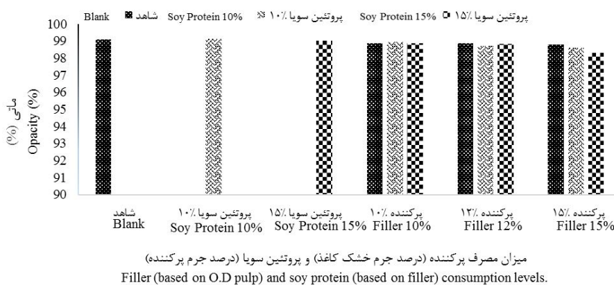
شکل ۶- تأثیر افزودن پرکننده و پروتئین سویا پیش‌اختلاط‌شده بر ماتی کاغذ.
