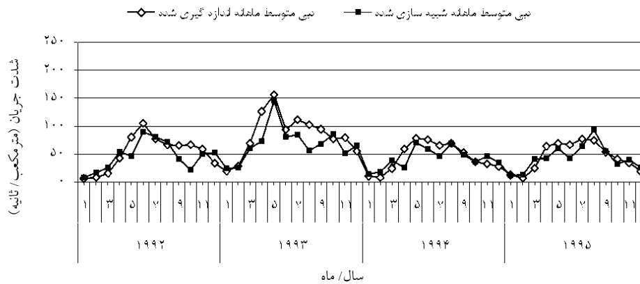
شکل ۴- نتایج واسنجی مدل در ایستگاه سد زاینده رود.
