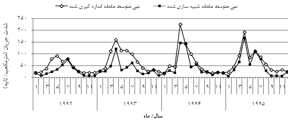
شکل ۳- نتایج واسنجی مدل در ایستگاه قلعه شاهرخ.
