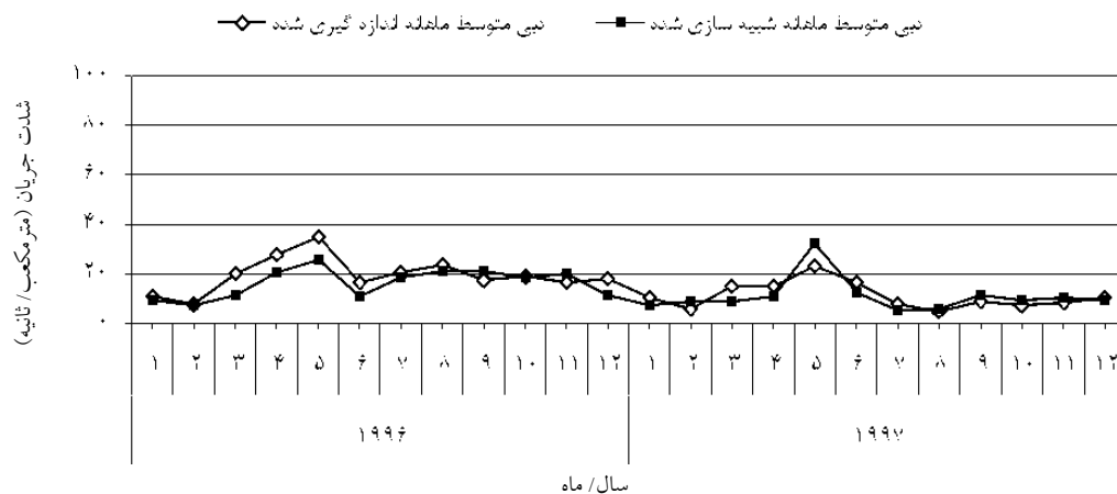
شکل ۷- نتایج اعتبارسنجی مدل در ایستگاه قلعه شاهرخ
