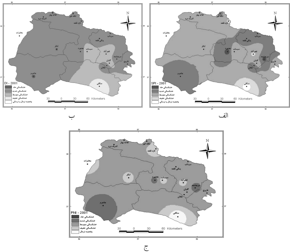
شکل ۲- پهنه‌بندی خشک‌سالی هوشناسی با استفاده از SPI (الف)، DI (ب) و PNI (ج) در استان خراسان شمالی در سال ۲۰۰۱.
