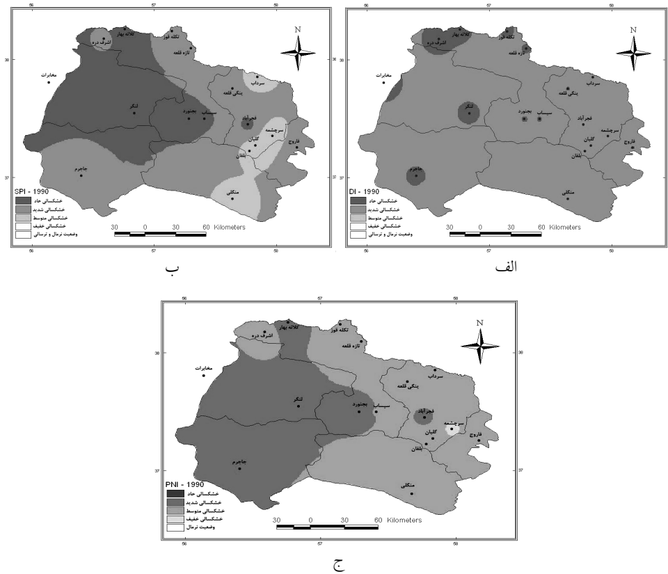
شکل ۱- پهنه‌بندی خشک‌سالی هوشناسی با استفاده از SPI (الف)، DI (ب) و PNI (ج) در استان خراسان شمالی در سال ۱۹۹۰.
