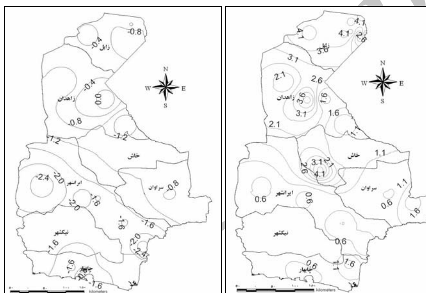
شکل ۵- پهنه‌بندی خشک‌سالی به روش کرجینگ با شاخص SPI برای ماه ۱۱ سال ۲۰۰۰ الف): مقیاس زمانی یک‌ماهه و ب): مقیاس زمانی ۱۲ ماهه.
