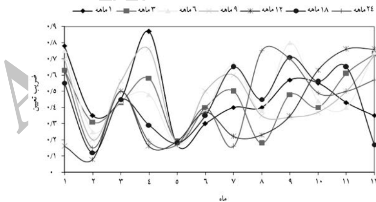
شکل ۴- مقایسه ضریب تعیین مربوط به روش کرجینگ با نیم‌تغییرنمای گوسی در ماه‌های مختلف برای سری‌های زمانی مختلف.
